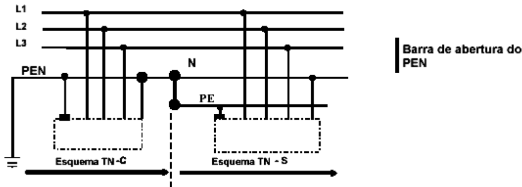
Esquema TN - C - S sem transformador de isolamento
