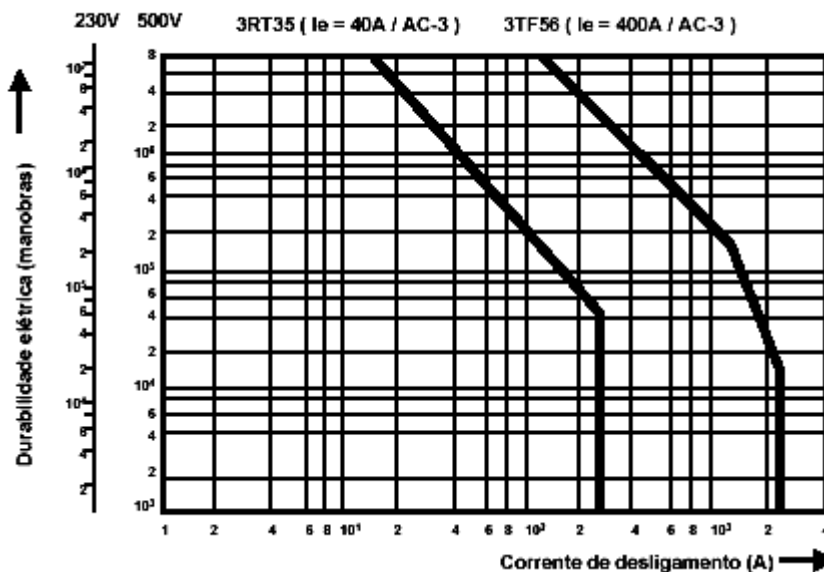
Durabilidade elétrica dos contatos.
