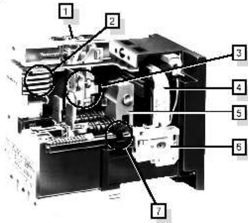
Contator de potência. Peça em corte.
